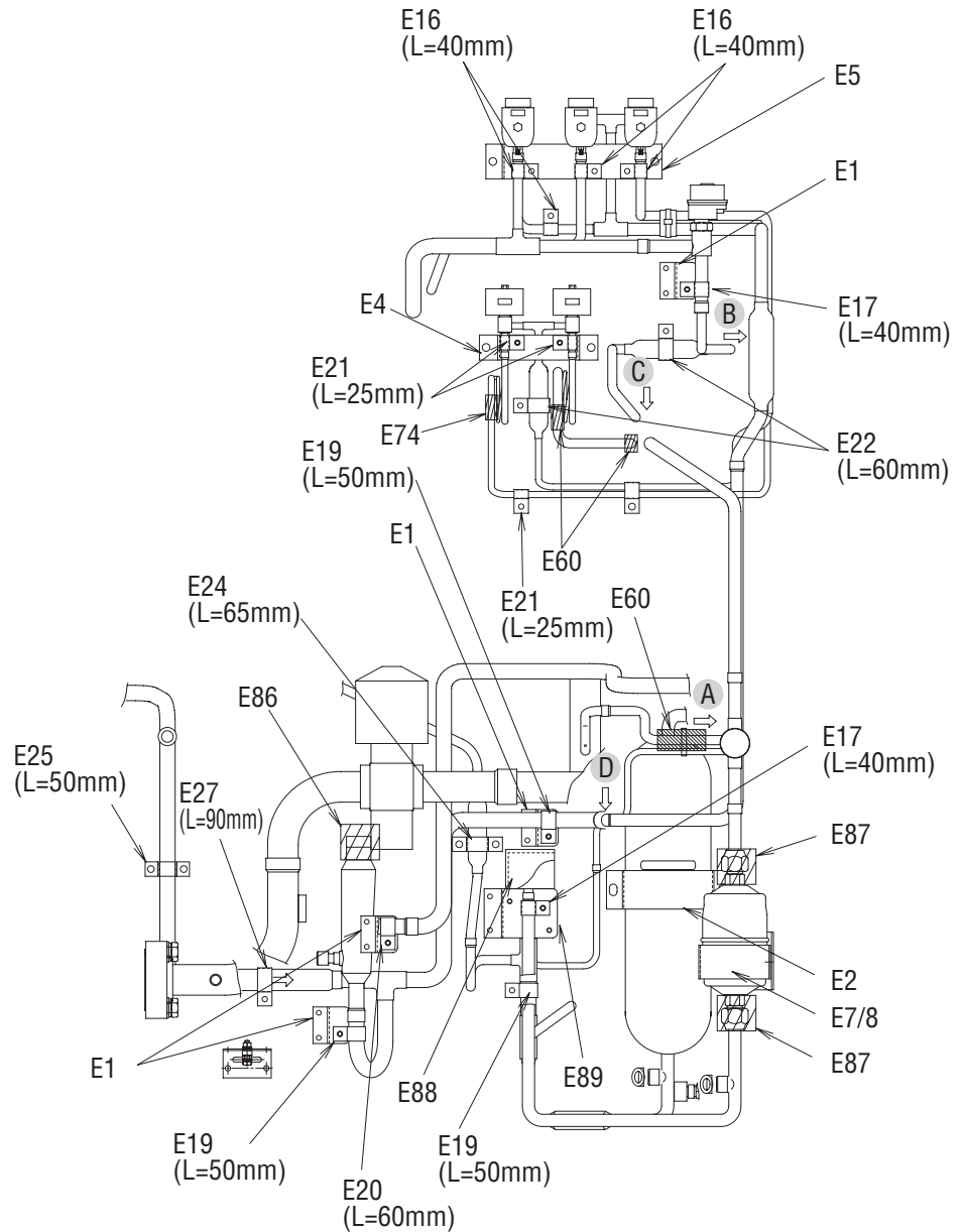
ドライヤー部詳細 (Dryer part detail)
